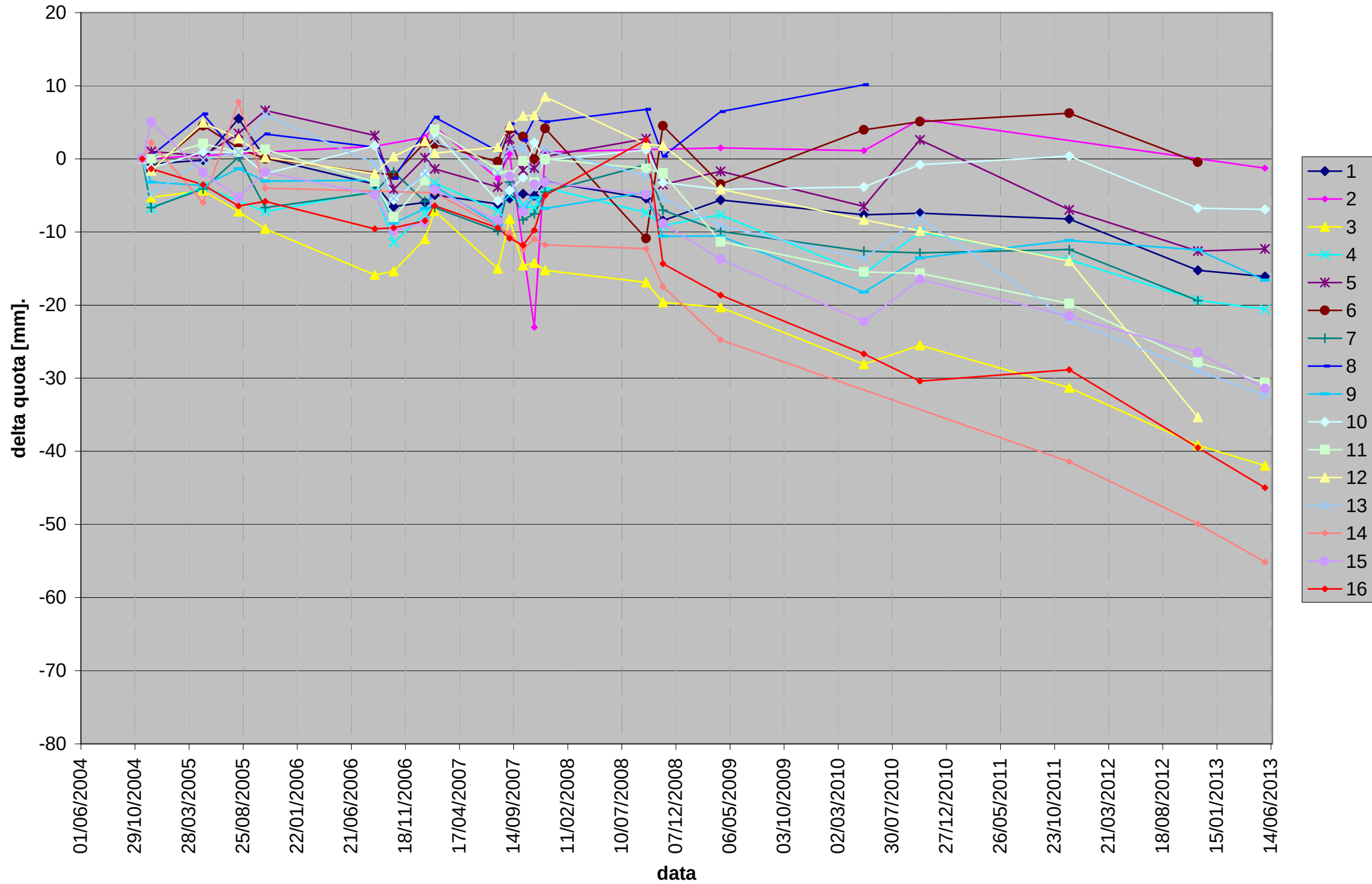
Villarendena OLTRESARCA - componente verticale
