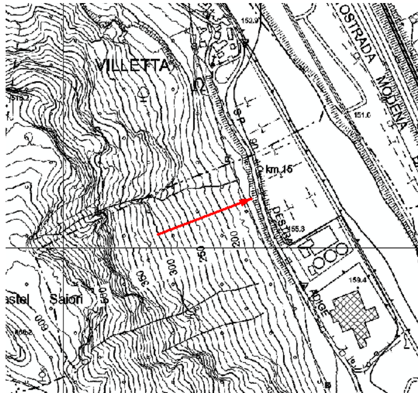
Figura 1: Corografia area del sopralluogo. La linea rossa indica la traiettoria dei blocchi.
